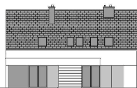
ELEWACJA OGRODOWA
