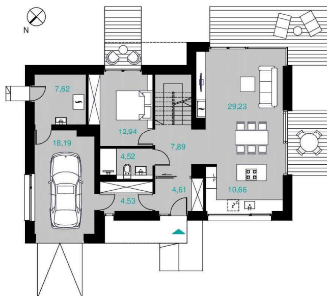
RZUT PARTERU 82,00 m 2 + GARAŻ 18,19 m 2
